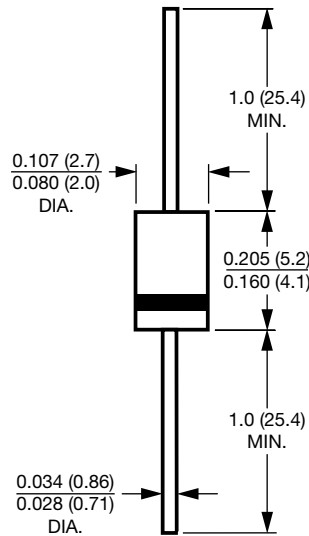
DO-204AL (DO-41)
