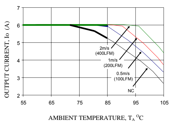
V_o=2.5V
